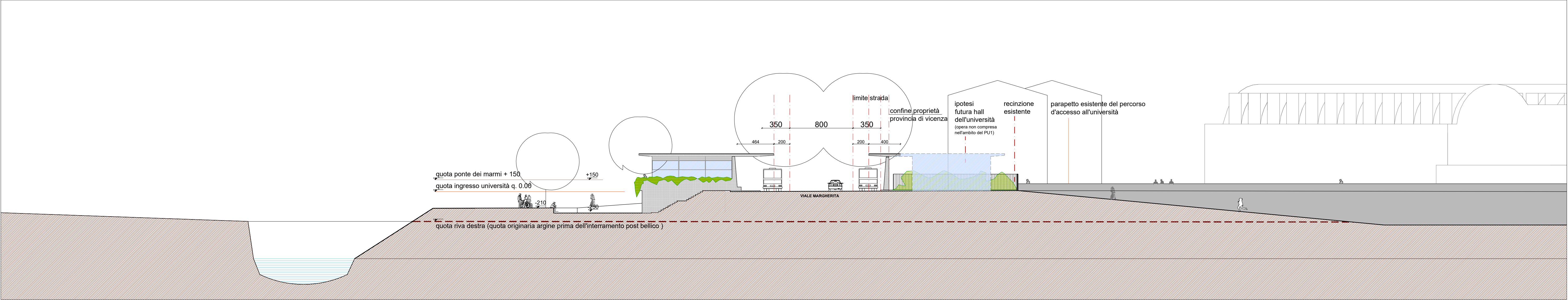
sezione AA
