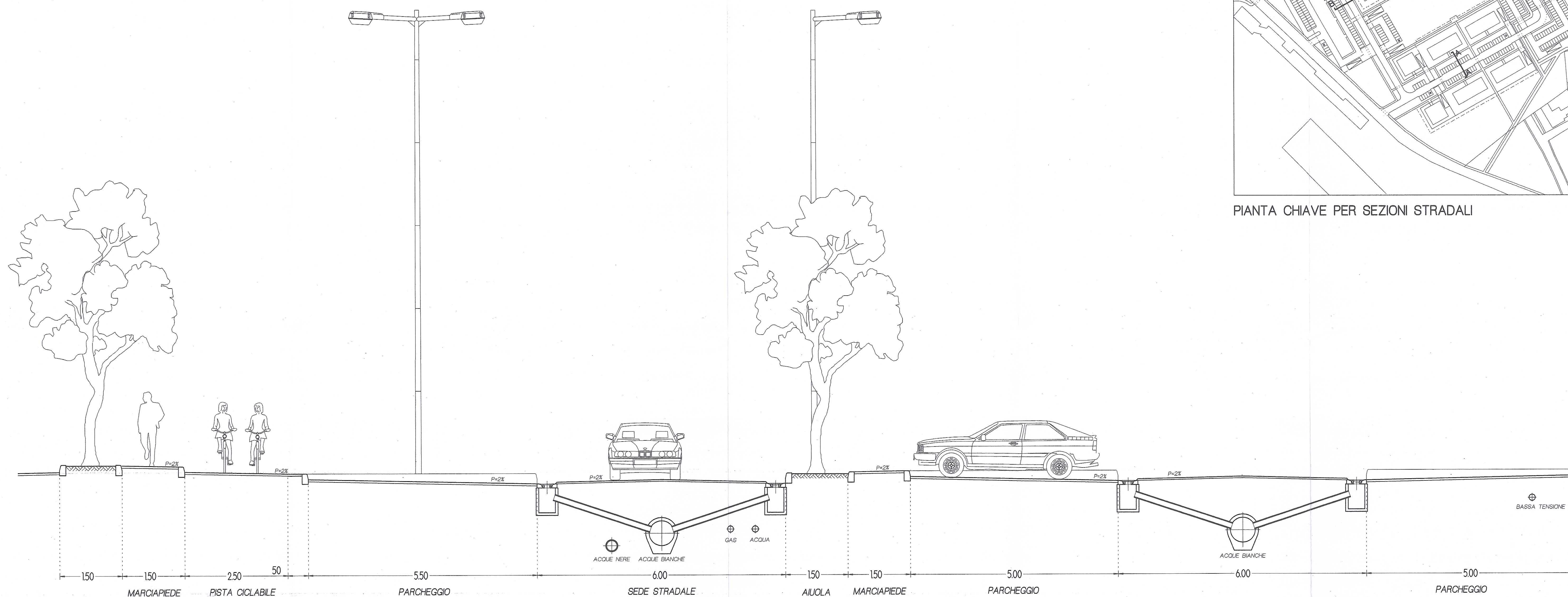
SEZIONE TIPO D-D
