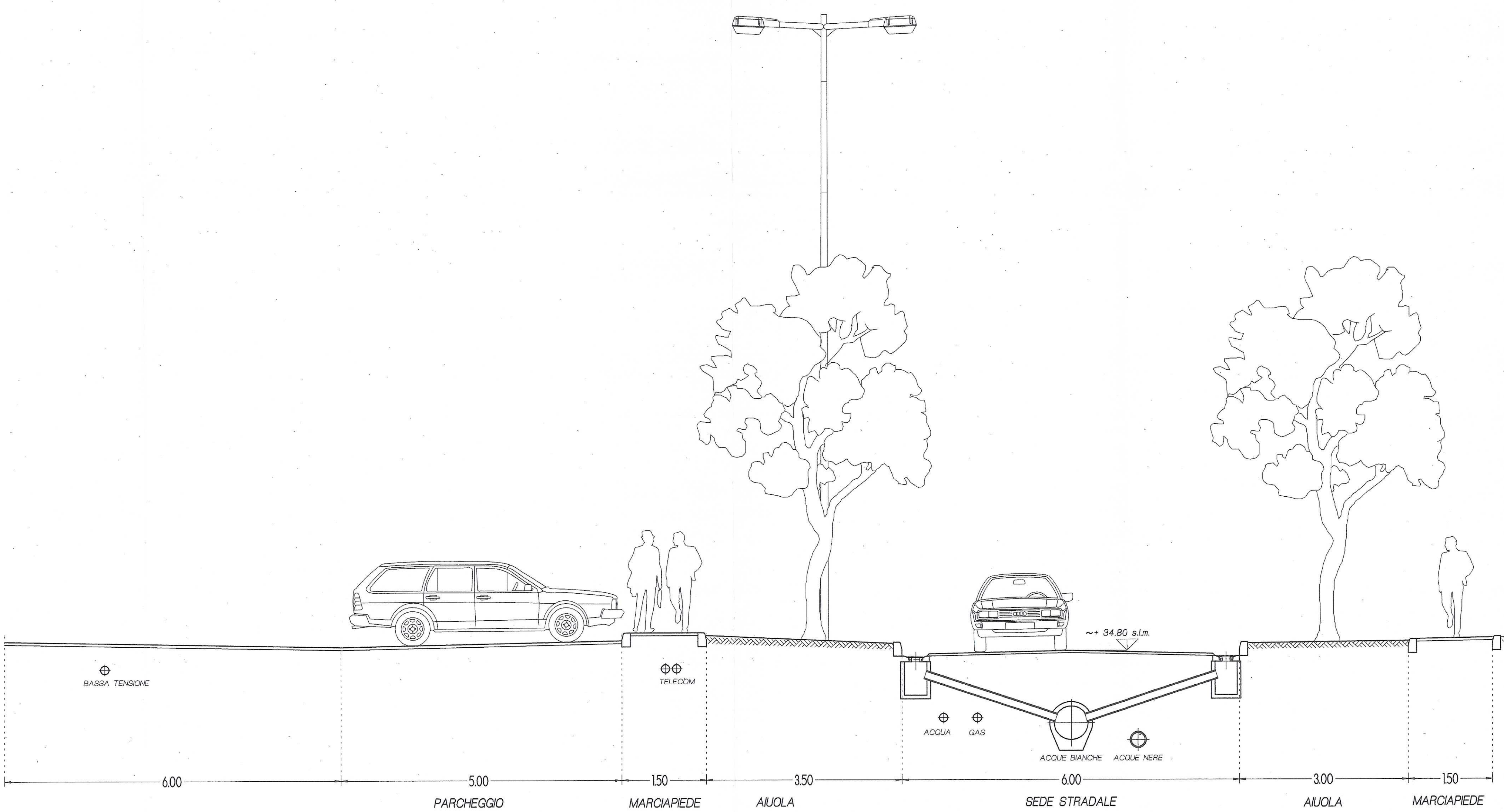
SEZIONE TIPO B-B
