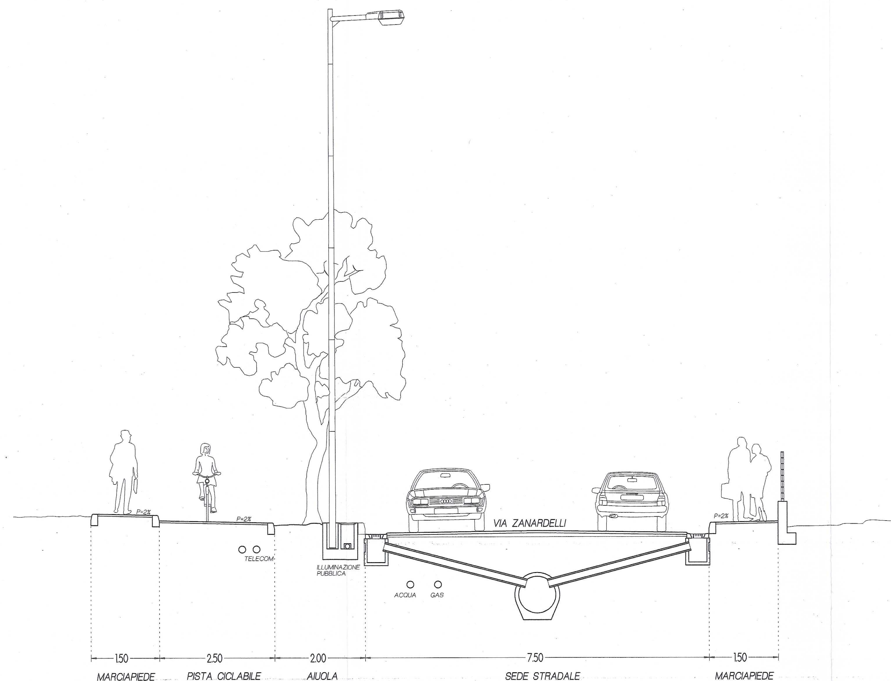
SEZIONE TIPO C-C
