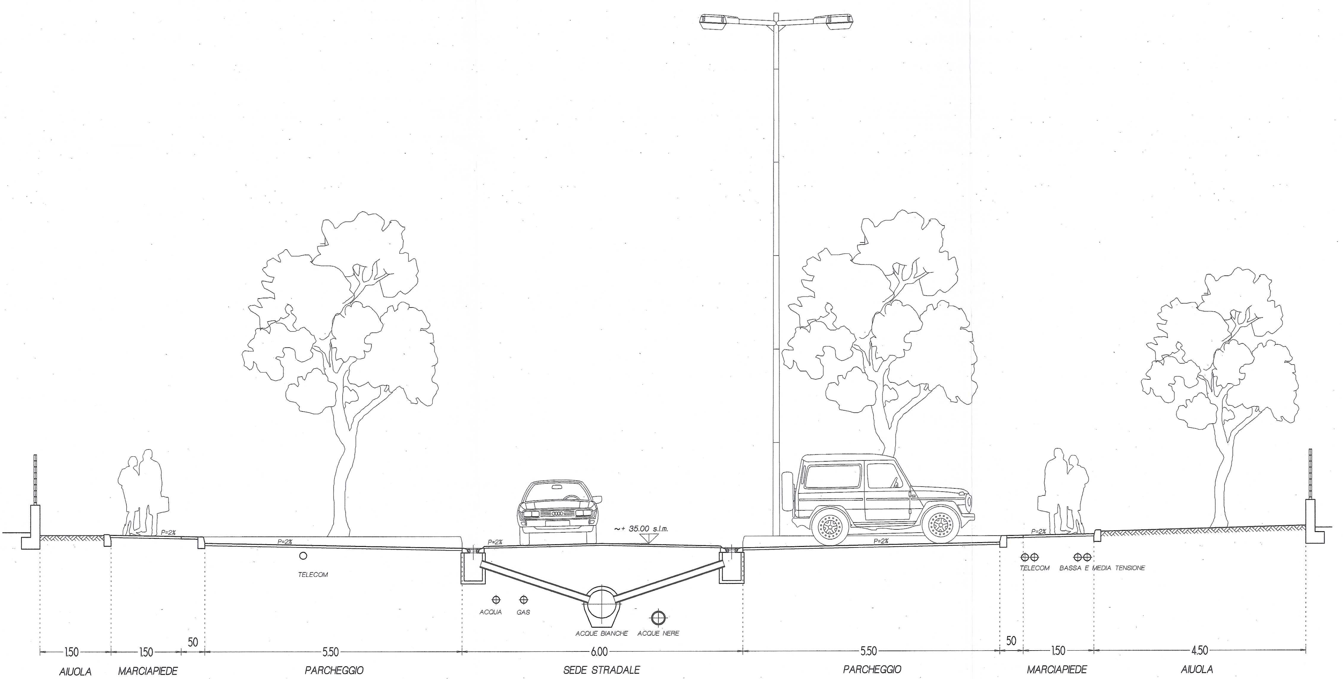
SEZIONE TIPO A-A
