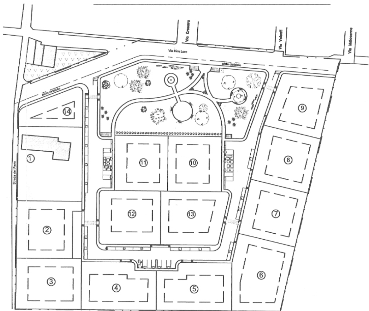
SISTEMAZIONE DEL VERDE AMBIENTALE scala 1 : 1000
