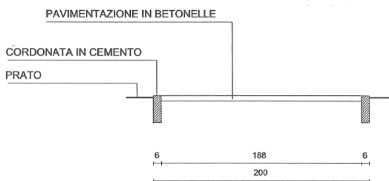
SEZIONE TIPO VIALETTO scala 1 : 20
