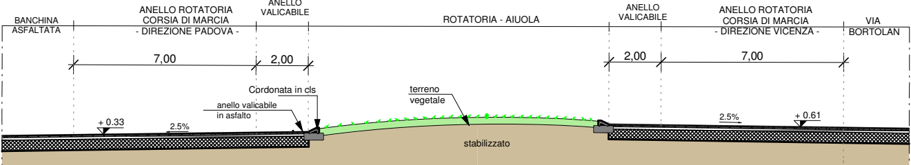
SEZIONE B-B 1:200
