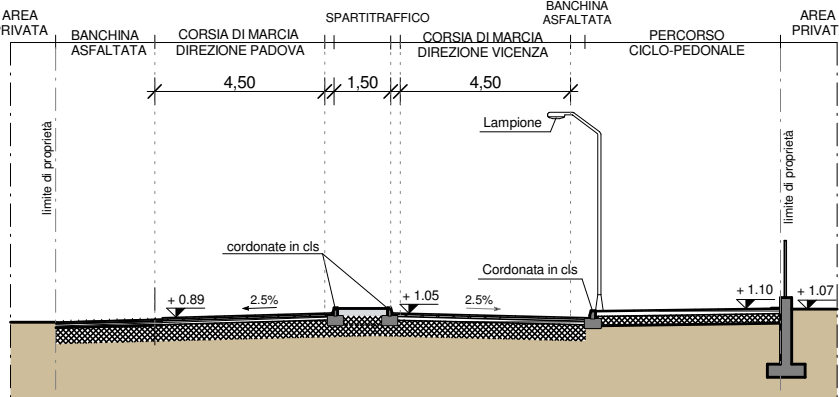
SEZIONE C-C 1:200
