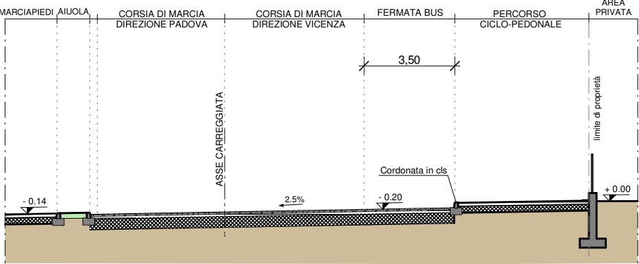
SEZIONE A-A 1:200
