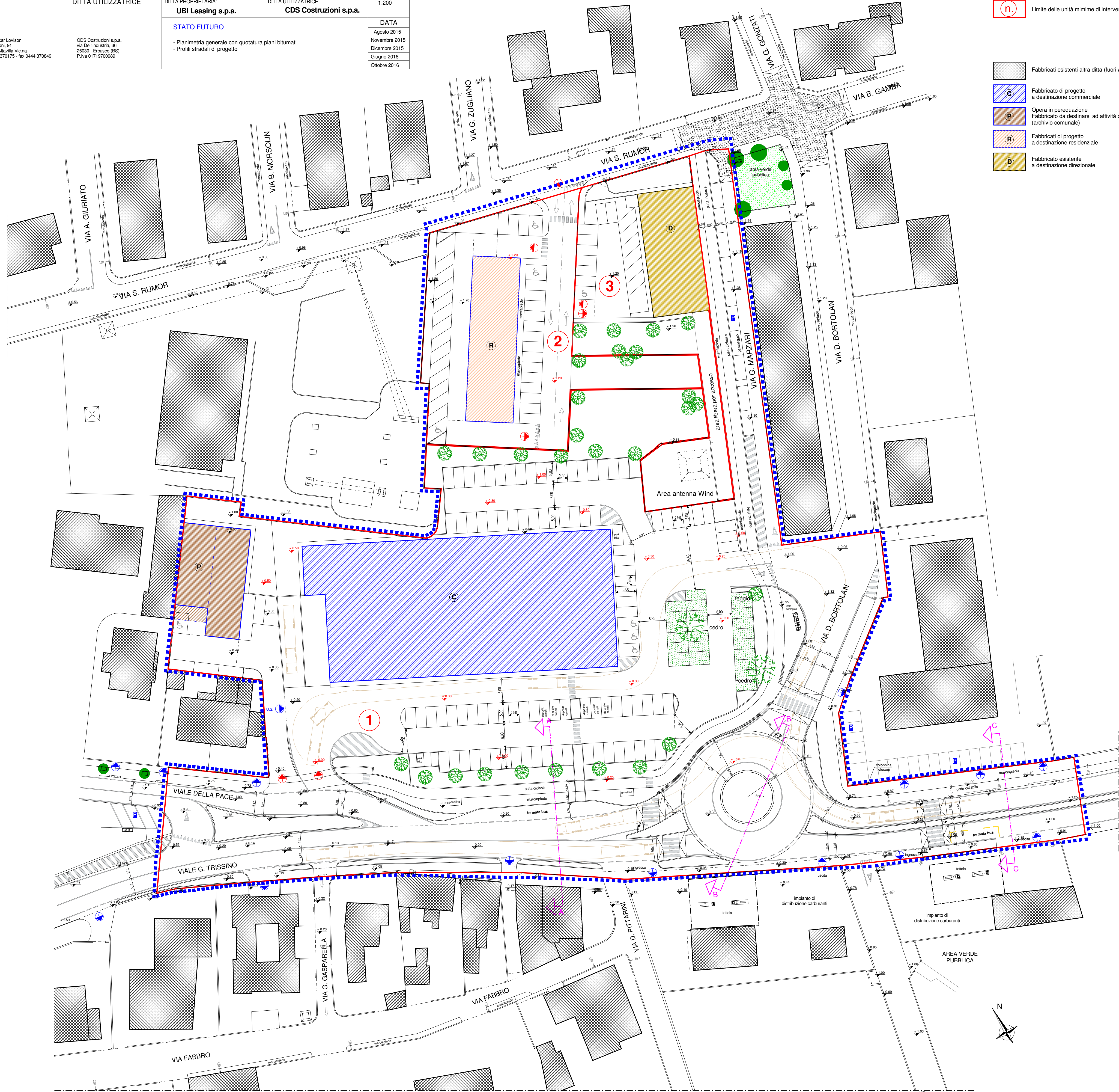
PLANIMETRIA GENERALE 1:500 - con quotatura piani bitumati
